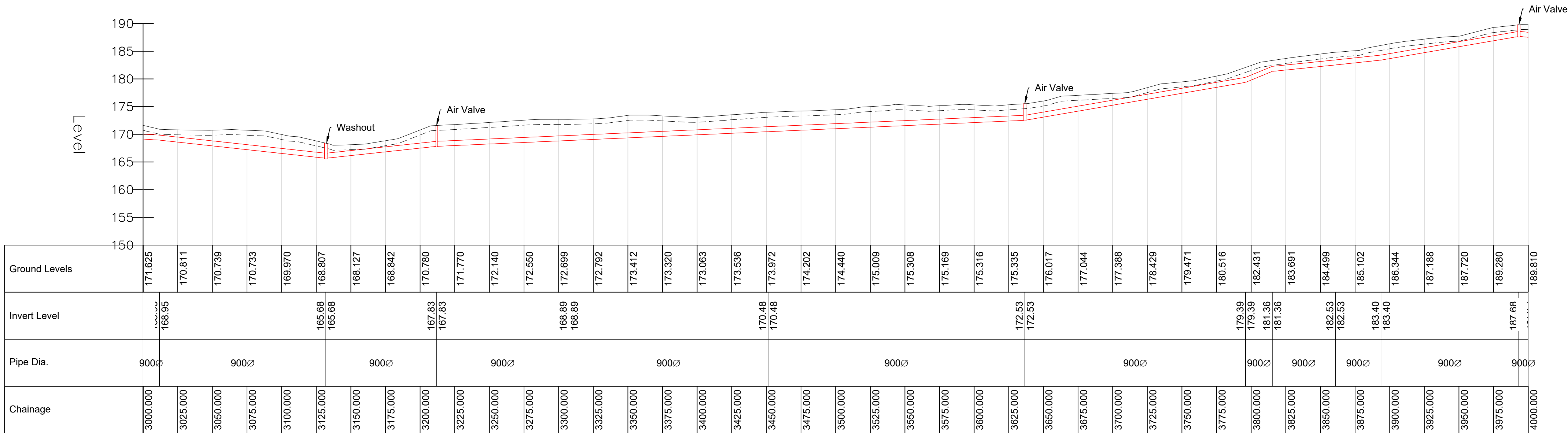
East Shaft - Reservoir (3000 - 4000m) Scale: H 1:2000,V 1:500. DATUM: 150.000
